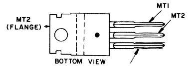
JEDEC TO-220AB
