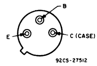
JEDEC TO-39
