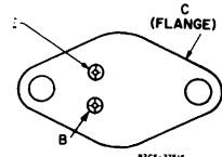
JEDEC TO-3
