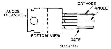
JEDEC TO-220AB
