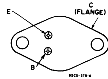
JEDEC TO-204MA
