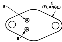
JEDEC TO-204MA
