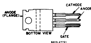
JEDEC TO-220AB
