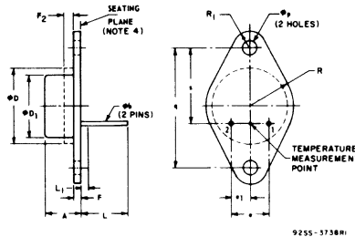
TO-213MA/TO-66
