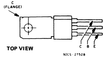
JEDEC TO-202AB
