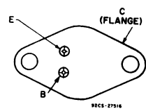
JEDEC TO-66
