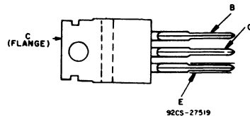
BOTTOM VIEW JEDEC TO-220 AB
