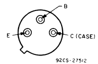
JEDEC TO-39 2N3439, 2N3440, 40346 40385, 40412
