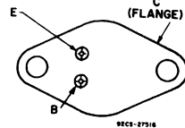
JEDEC TO-3
