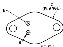
JEDEC TO3/TO-204MA
