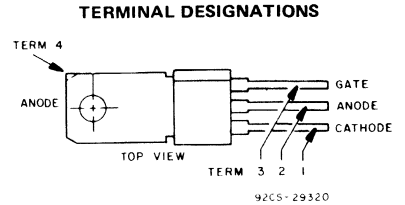
JEDEC TO-202AB
