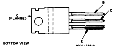
JEDEC TO-220AB
