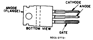
JEDEC TO-220AB
