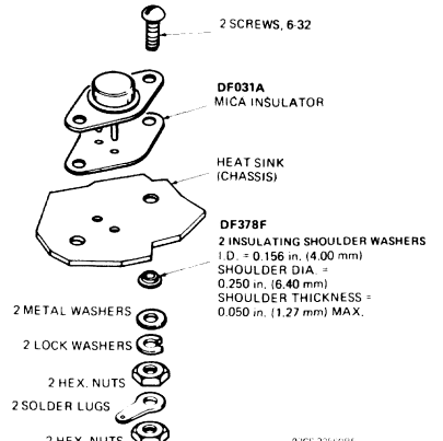
TO-213MA/TO-66
